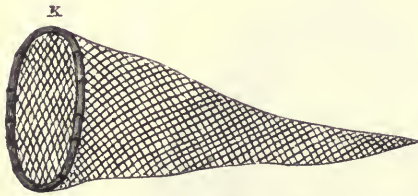
200. ábra. Szádellői farkasháló.
