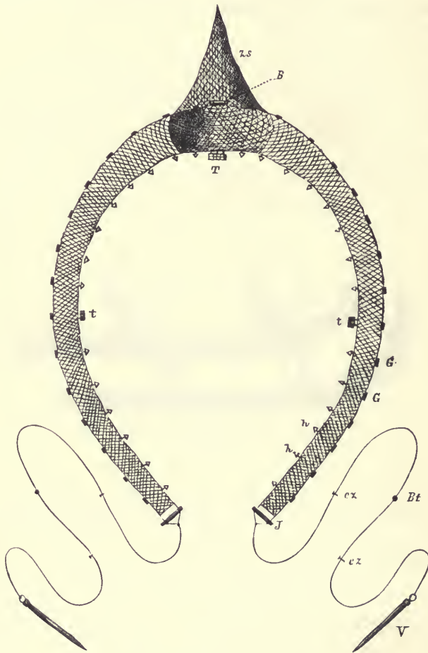
265. ábra. Öregháló jeges halászátra.
